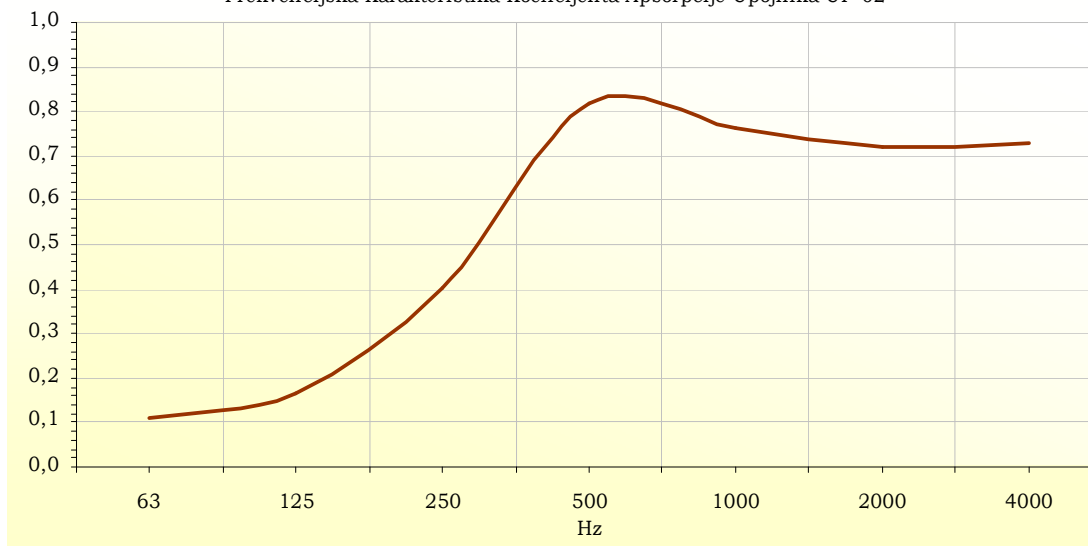
Frekvencijska Karakteristika Koeficijenta Apsorpcije Upojnika UP-02
